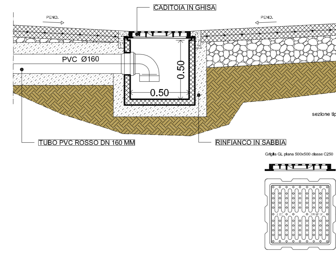
Particolare: caditoia scala 1:20
