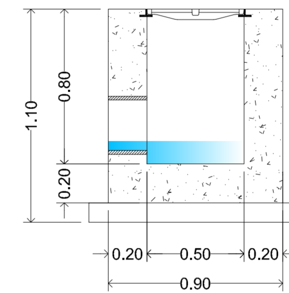
Particolare: canaletta con griglia scala 1:20
