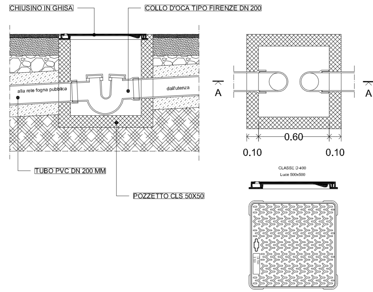
Particolare: pozzetto sifonato scala 1:20
